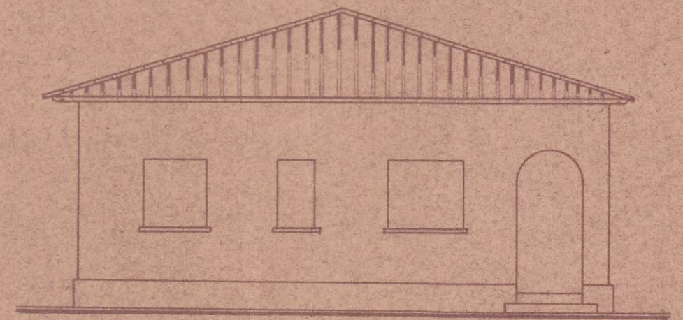
Fachada Oeste.
