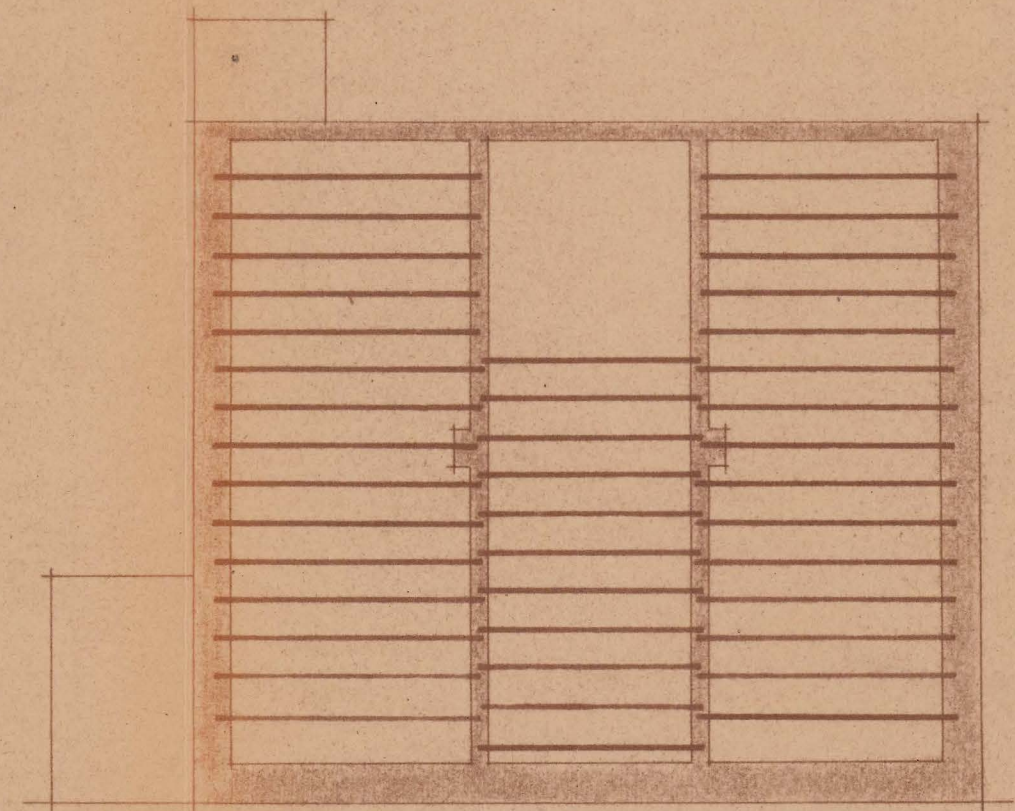
entramados de piso
