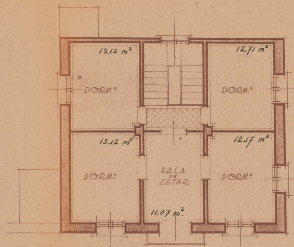
planta 1ª
