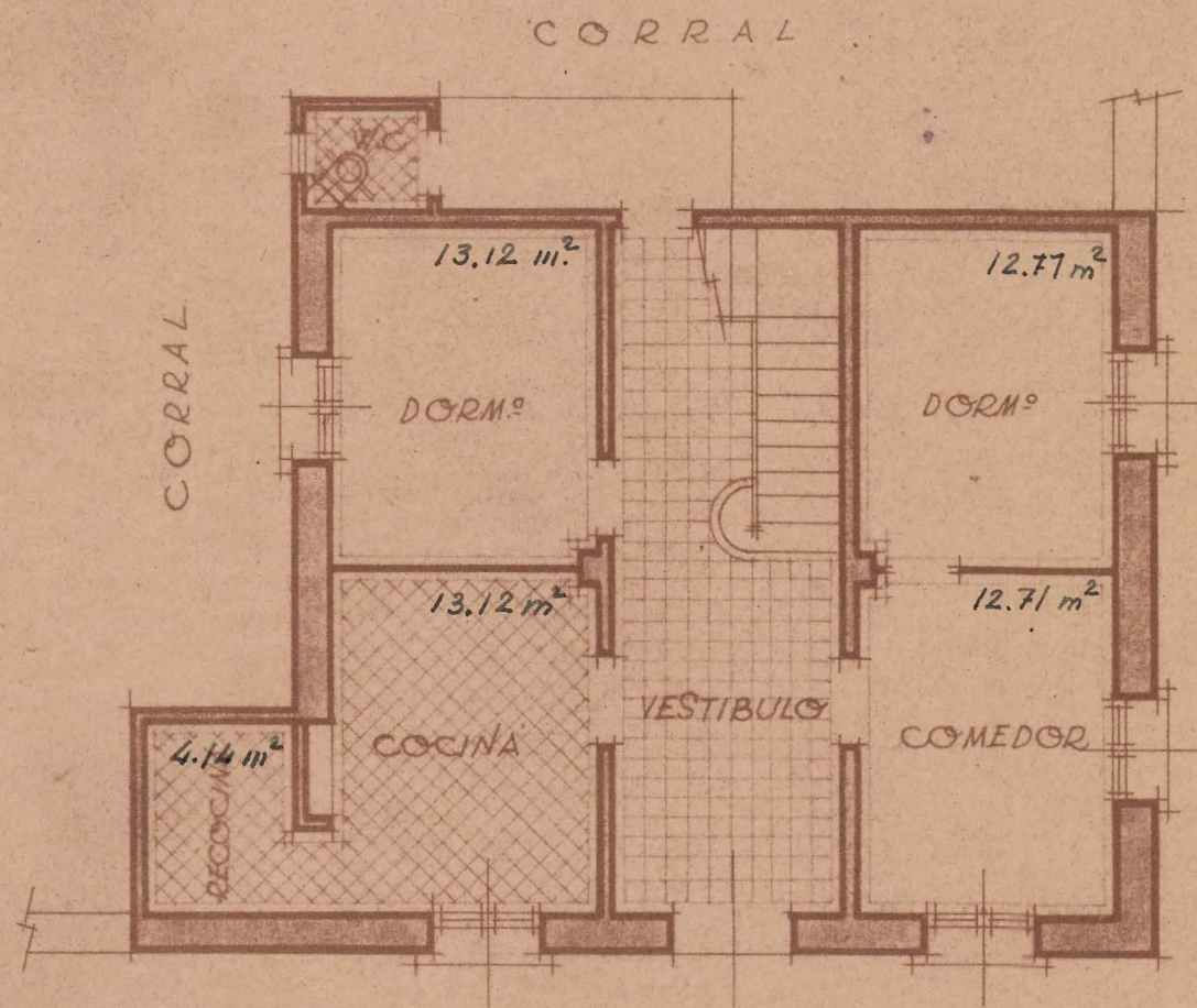
planta baja
