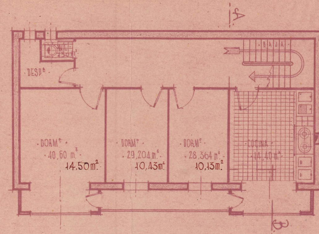
PLANTA PISO 1º
