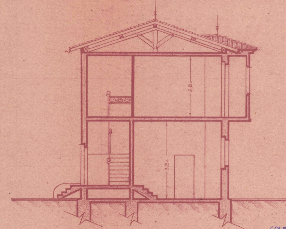
SECCION A-B
