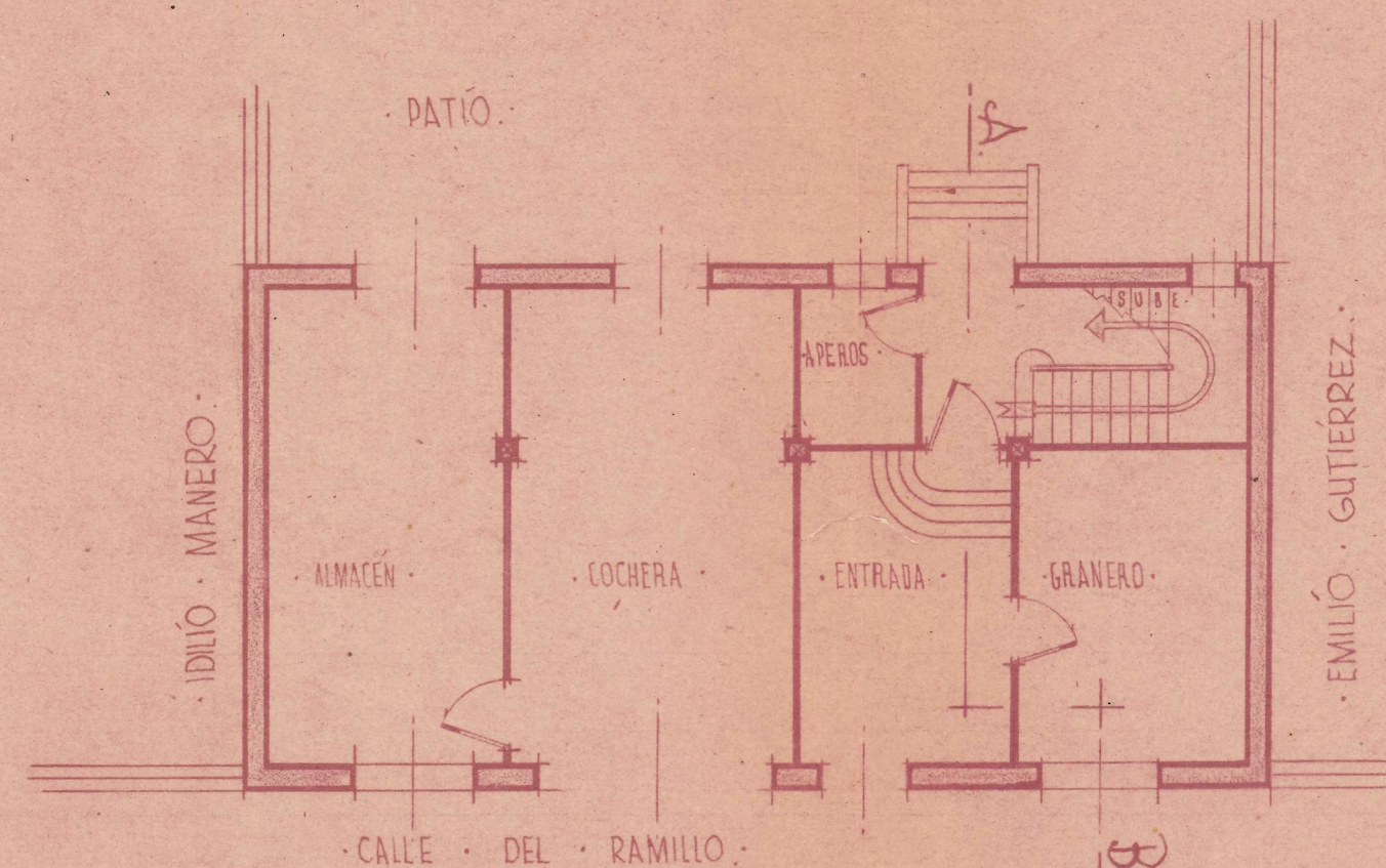
PLANTA BAJA
